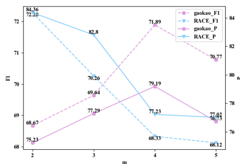
图 5. 筛选模块中m值变化
