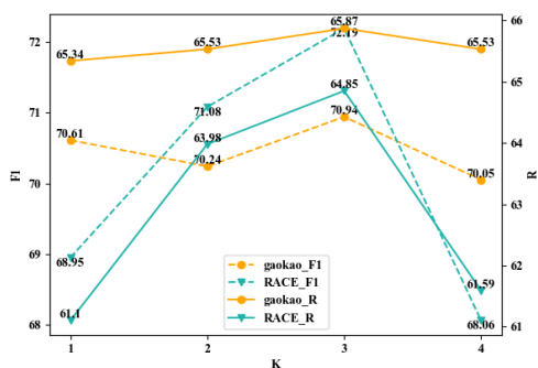
图 4. 递归抽取中K值变化
